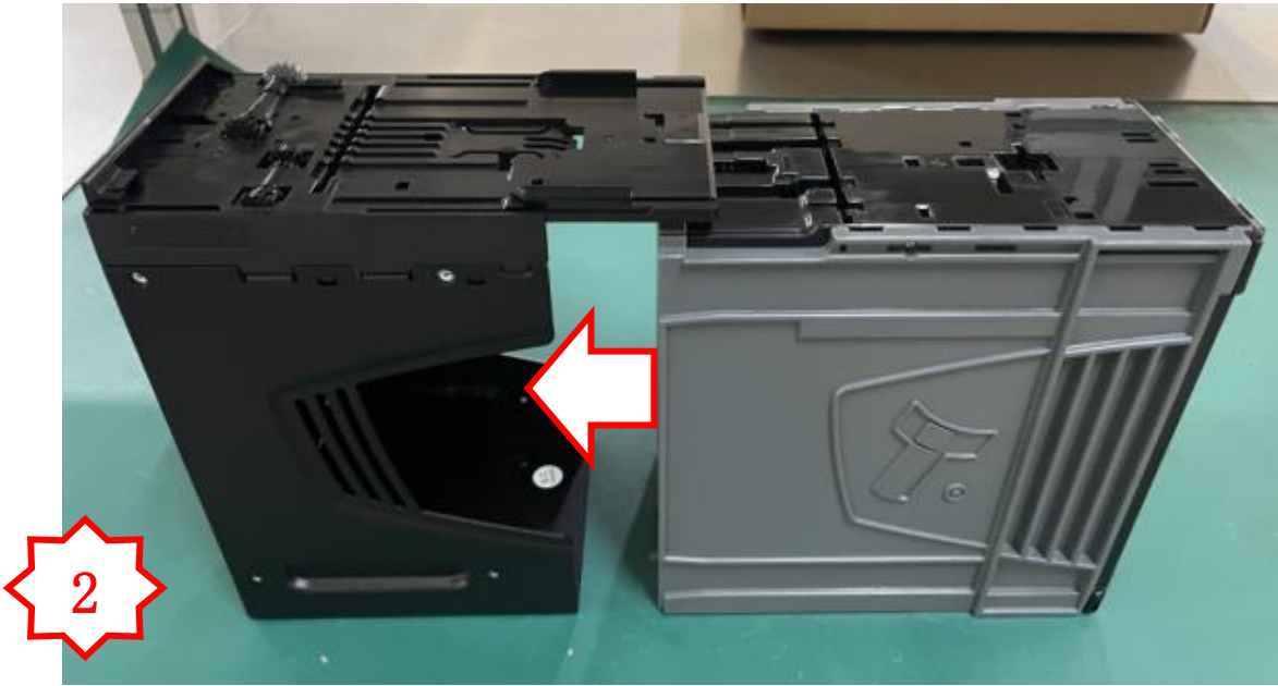
图二，将 NV200ST CB1000 V2 内箱推入 NV200S 外箱
