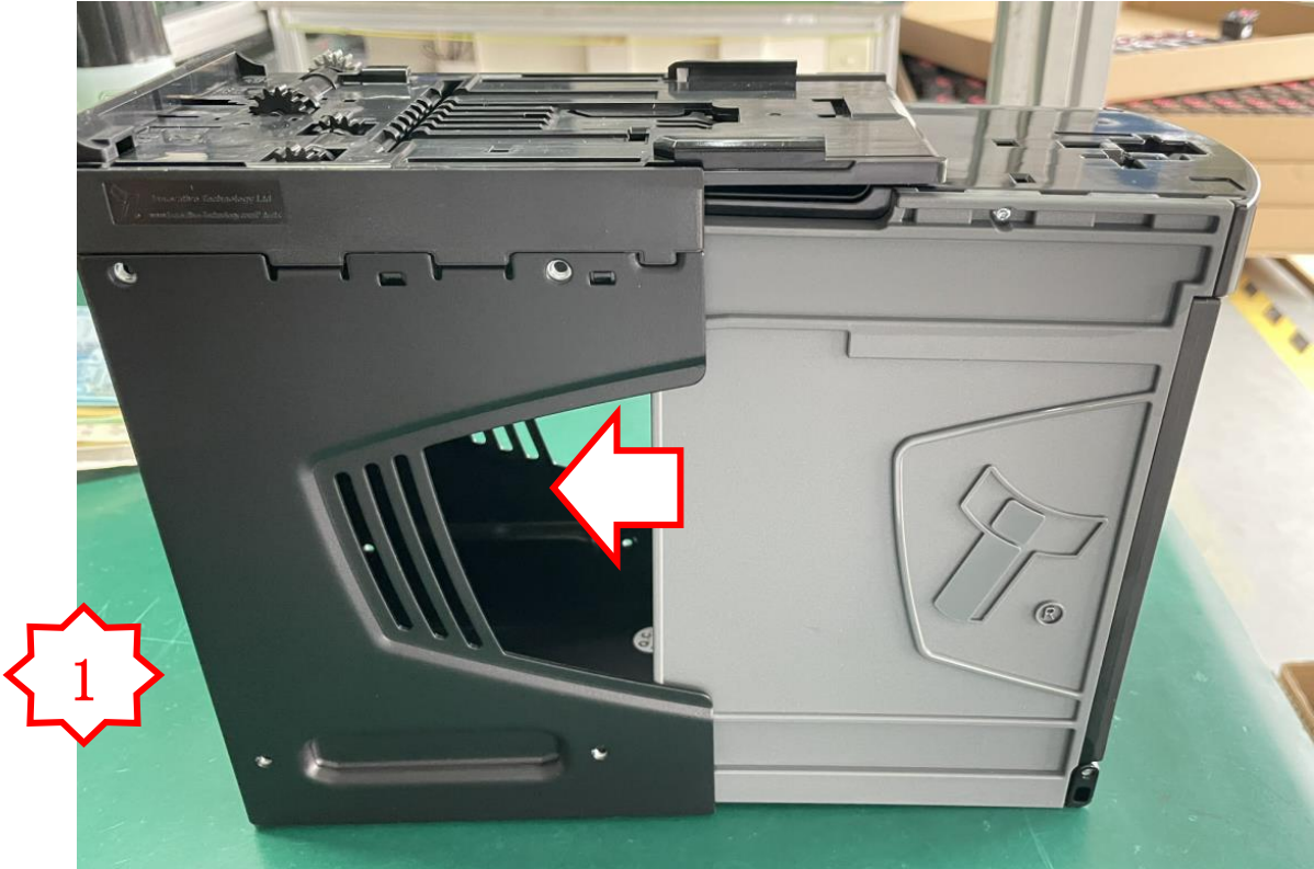
图一，将 NV200ST CB500 V2 内箱推入 NV200S 外箱
